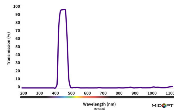
BP450 INDIGO BANDPASS
